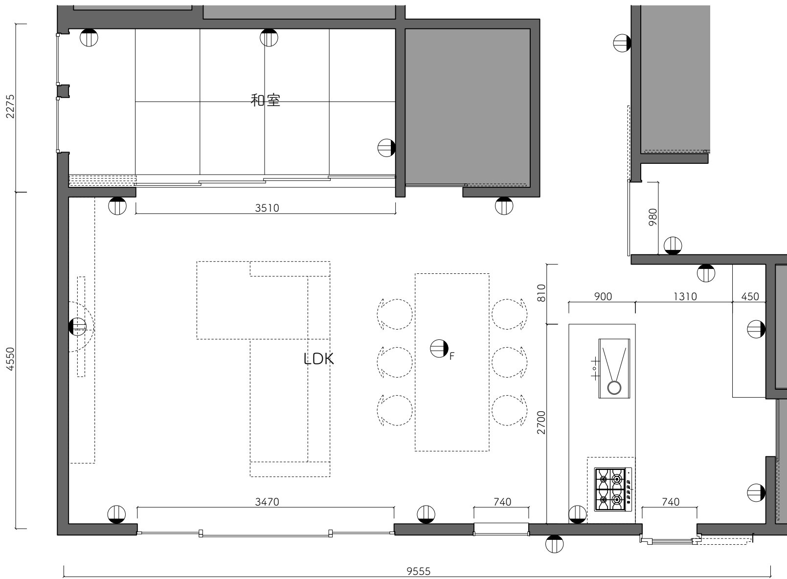
1階平面詳細図 1/50 on A4
